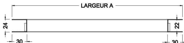
coupe horizontale
