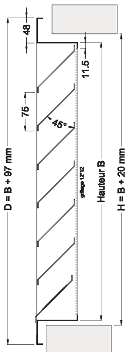
coupe verticale
