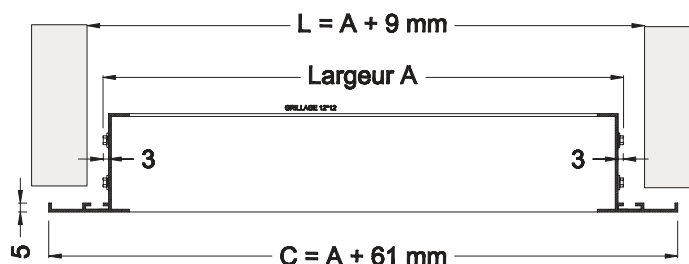
coupe horizontale
