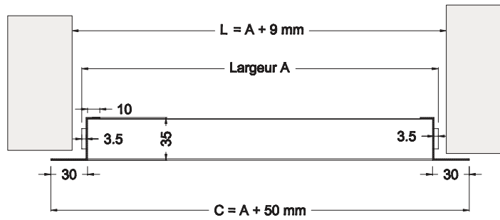
coupe horizontale
