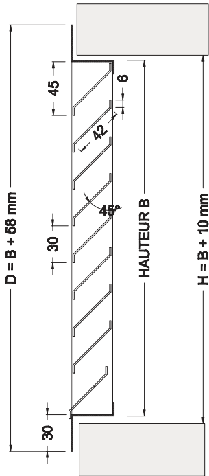
coupe verticale
