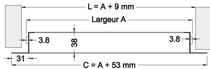
coupe horizontale
