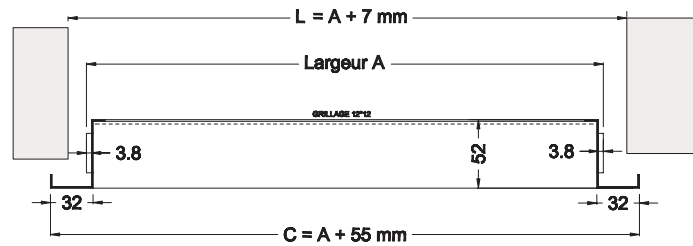
coupe horizontale
