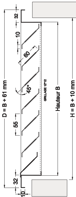
coupe verticale
